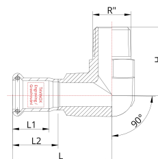
Technický náčres
