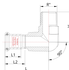
Technický náčres
