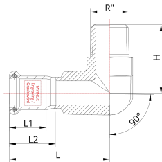
Technický náčrt
