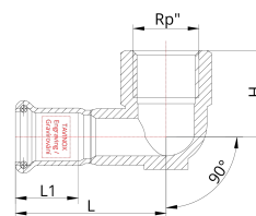
Technický nákres
