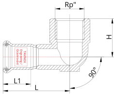
Technický nákres
