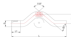
Technický náčrt
