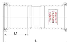
Technický náčres
