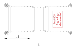
Technický náčres
