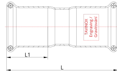
Technický náčres
