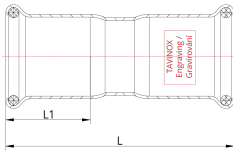
Technický náčres
