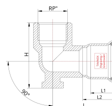
Technický náčrt
