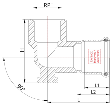
Technický náčres
