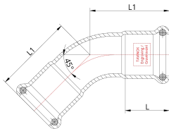
Technický náčres
