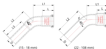
Technický náčrtek
