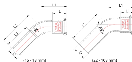
Technický náčrt
