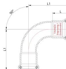
Technický náčrtek
