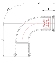
Technický náčres
