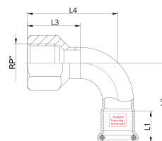
Technický náčrt
