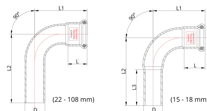
Technický náčrt
