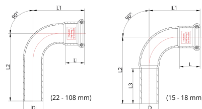
Technický náčres
