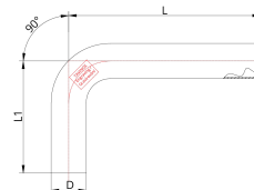
Technický náčres
