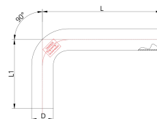
Technický náčres
