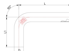
Technický náčres
