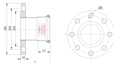
Technický náčrt
