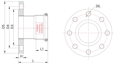
Technický nákres
