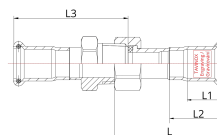
Technický náčrt
