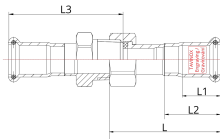
Technický náčres
