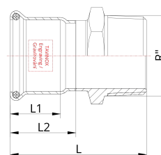
Technický náčres
