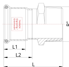
Technický náčes
