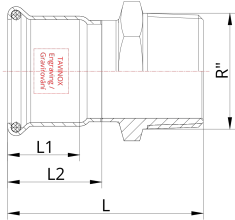
Technický náčrt
