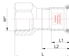
Technický náčes
