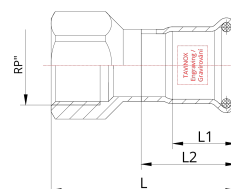
Technický náčres
