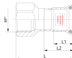
Technický náčes
