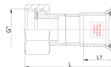
Technický náčrtek
