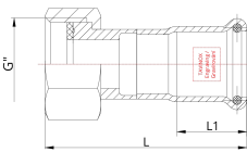
Technický náčres
