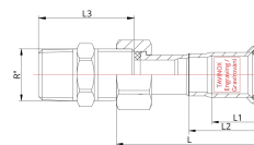
Technický náčres
