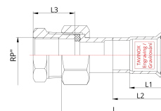
Technický náčres
