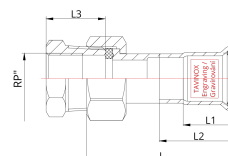
Technický náčres
