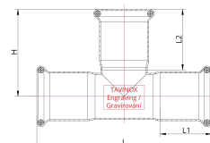
Technický náčrtek
