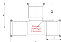
Technický náčrtek
