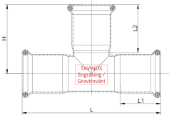
Technický náčres
