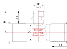
Technický náčres
