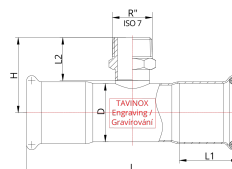
Technický náčres
