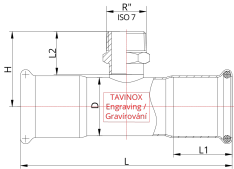
Technický nákres
