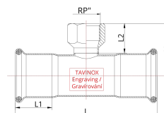
Technický náčrt
