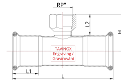
Technický náčrt
