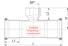
Technický náčrt
