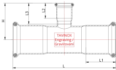
Technický náčrt
