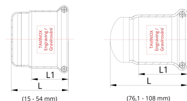
Technický náčres
