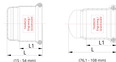
Technický náčres
